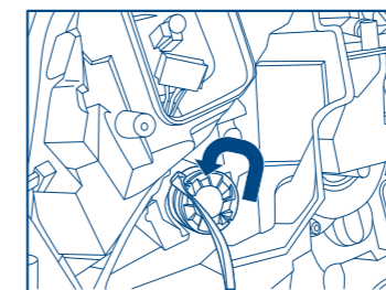
3 Scoateți inelul central și introduceți-l în suport. Fixați inelul cu clema metalică. Introduceți becul în suport. Răsuciți ușor becul pentru a-l fixa.
